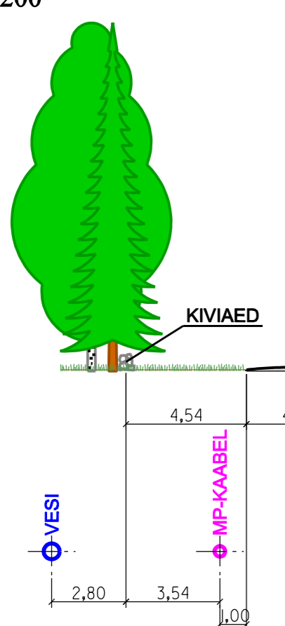
LÕIGE 1-1 M 1:200
