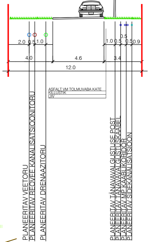
PLAN. SISETEE A-A
